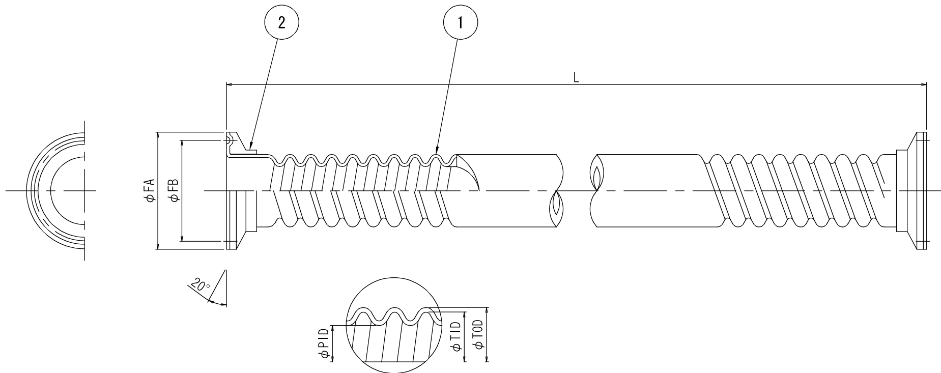
チューブ詳細
