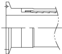
※1.0S、1.25Sフェルール形状
